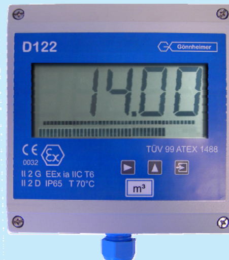
Digitales Anzeigegerät D122.A.7.x.x
